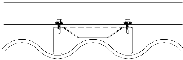
Figur 5.12 Stödbricka ovanför befintlig läktrad ställs ovanpå eternitskiktet.
