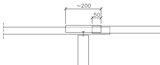
KOMBILÄKTENS ÄNDE KAPAS OCH SKJUTS ÖVER 50mm
