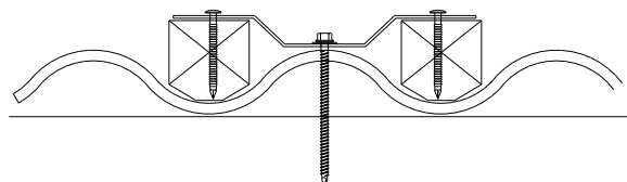
Figur 5.6 Infästning av träregel till låsbricka.
