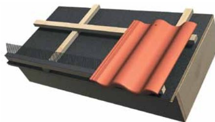
Bild 14. Fågelbandet monteras vid takfoten för att förhindra att fåglar bygger bo under takpannan. Det finns även ventilerat fågelband, används för tak med takfotskil.
