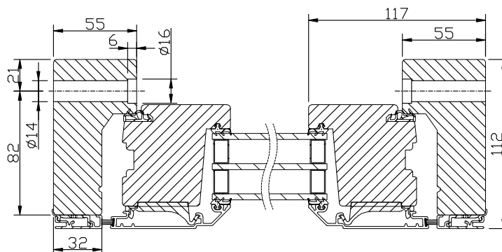
Horizontalsnitt
