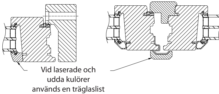
Horizontalsnitt pardörr
